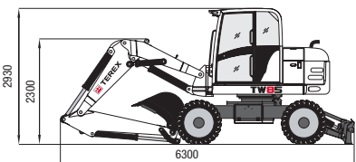
Abb. 3: Transportstellung
